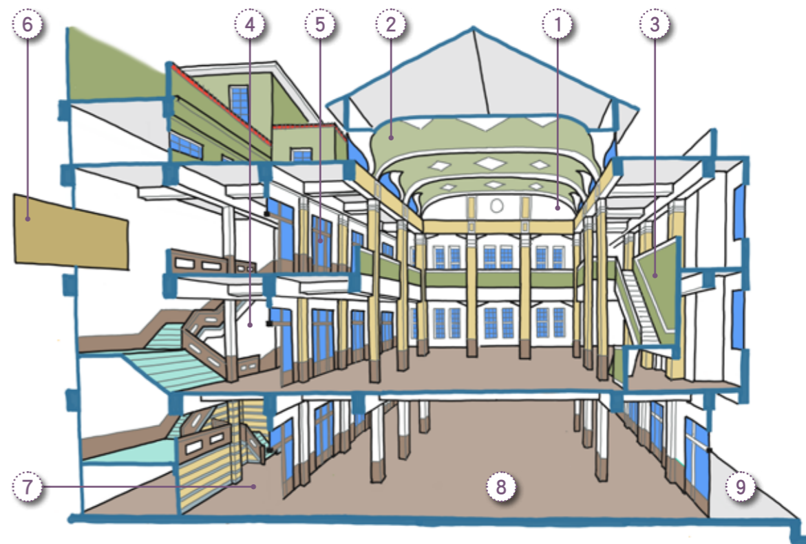
圖五 臺北公會堂大宴會廳(光復廳)剖面
